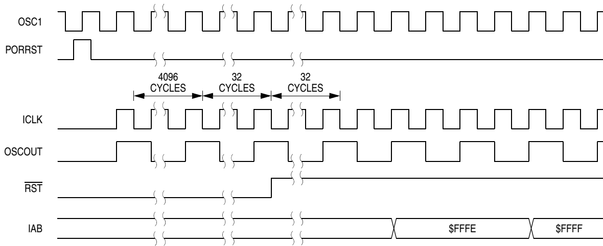
Figure 5-7. POR Recovery
