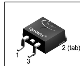
P- TO263 -3-2
